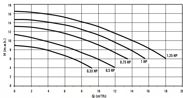
Prestandakurvor
