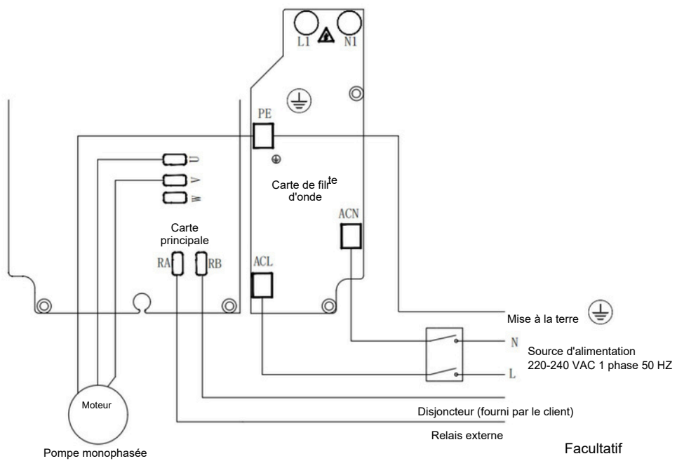
Fig. 6 Schéma de câblage pour pompe monophasée
