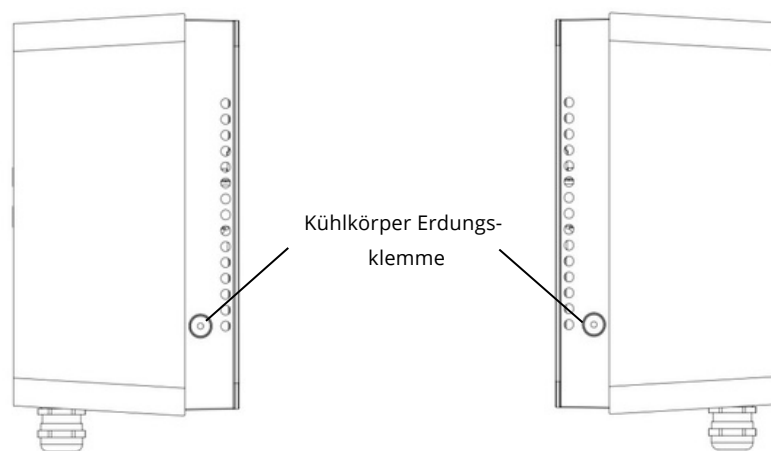
Abb.5 Erdungsleiter-Anschlusschema
