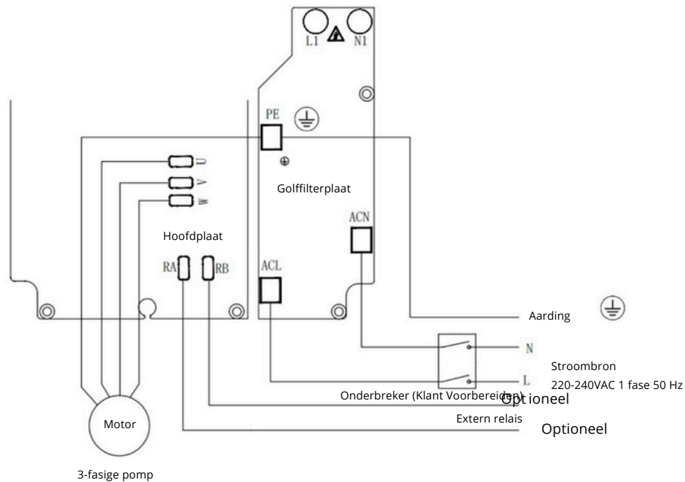
Fig 7 3-fase aansluitdiagram pomp
