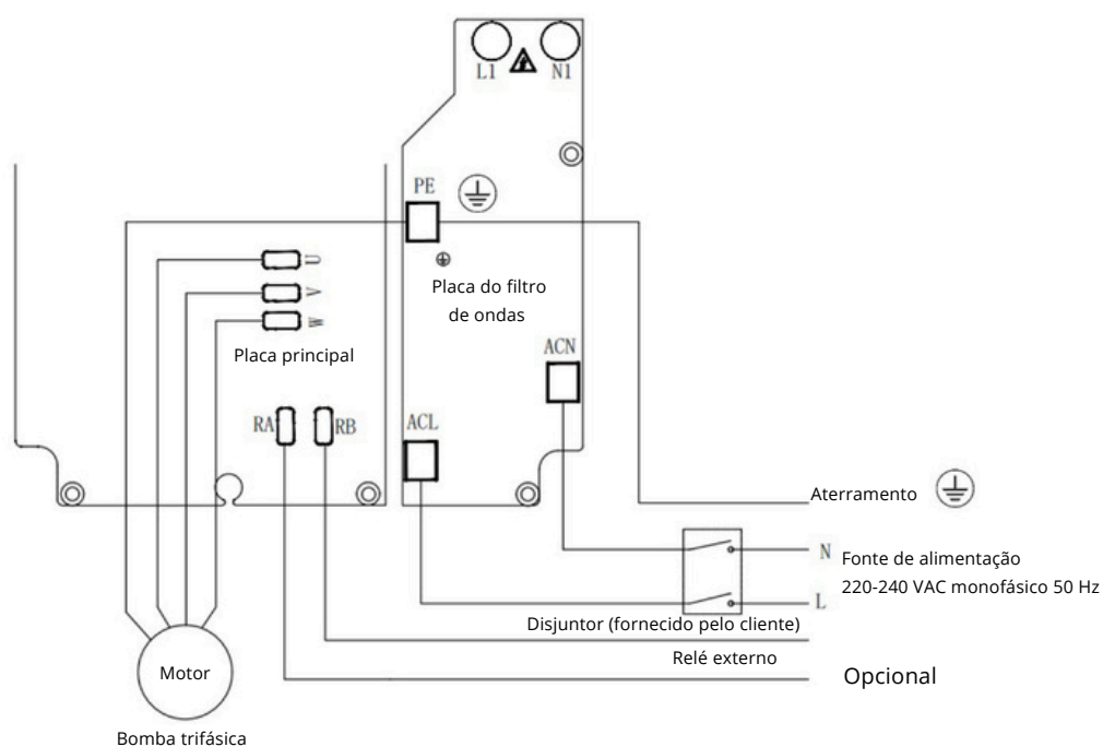
Fig. 7 Diagrama de ligação trifásica da bomba
