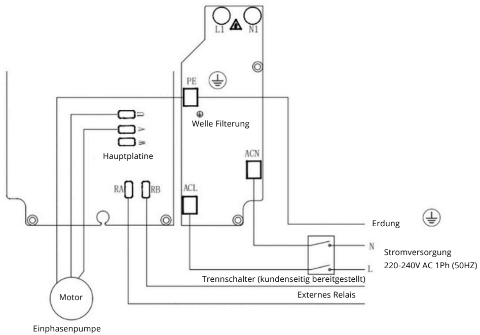
Abb. 6 1-ph Pumpenanschlussschema
