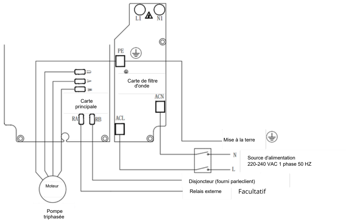
Fig. 7 Schéma de câblage pour pompe triphasée
