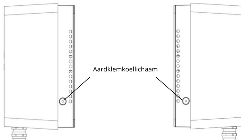
Fig.5 Aansluitschema aardingsdraad
