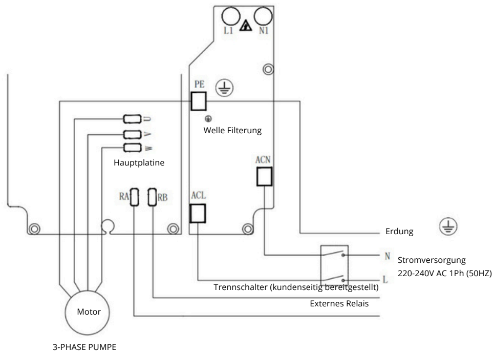
Abb. 7 3-ph Pumpenanschlussschema
