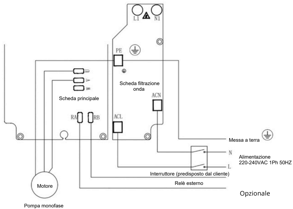
Fig. 6 Schema di collegamento della pompa monofase
